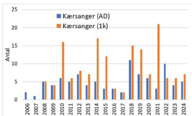
Figur 21a. Antal Kærsanger ringmærket og aflæst i perioden 2006-2024.
